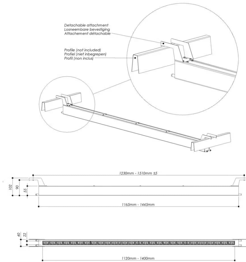
Lichttechnische tekening
